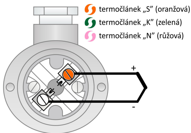
Obrázek 11F.6: Zapojení jednoduchého termočlánu
