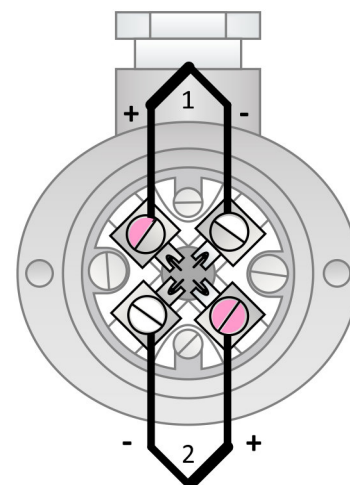
Obrázek 11F.7: Zapojení dvojitého termočlánu
